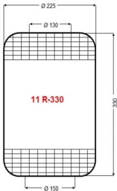
CONTITECH 1415N Zastosowanie: Iris Bus Citelis
