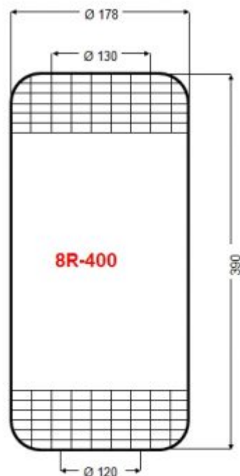
VOLVO 3111277, DUNLOP FA31095 Zastosowanie: Volvo
